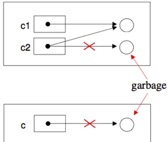
Figura 2.2: Gestione Memoria in Java.
