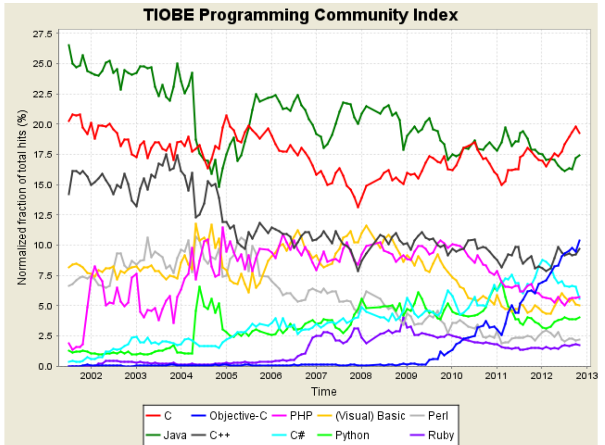
Figura 2: Linguaggi di programmazione più usati
