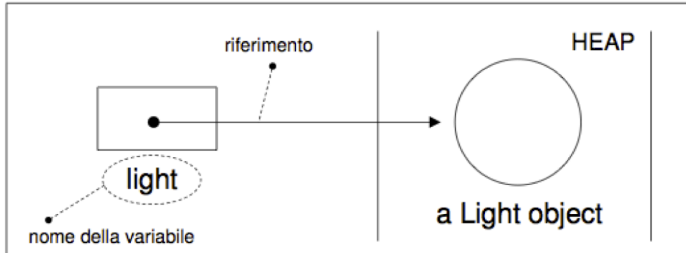
Figura 2.1: Gestione Memoria in Java.
