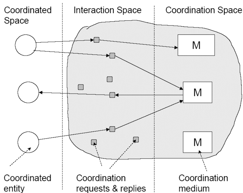
Figure 2.1: Architettura logica
