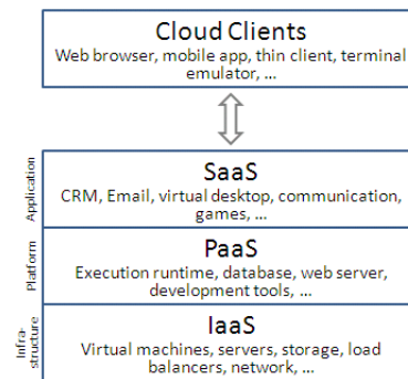
Figure 1.1: visione distribuzione Cloud
