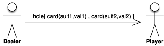
Fig. 9. Preflop state
