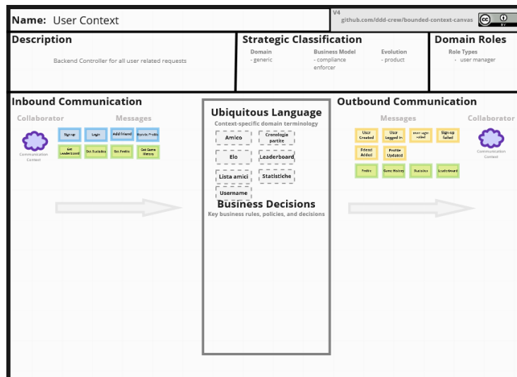
Figure 19: Bounded Context Canvas relativo all'utente
